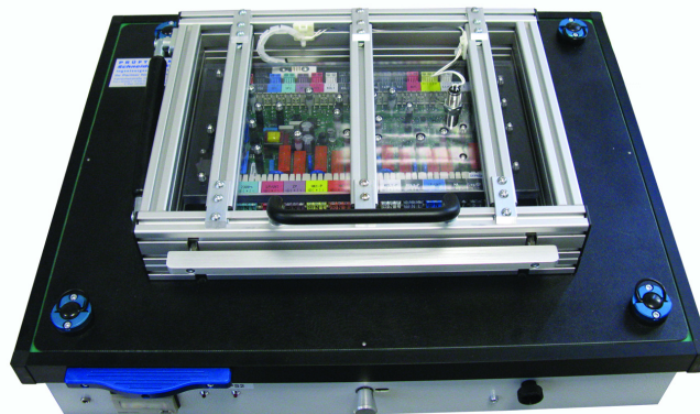
Abb. Schneider & Koch Vakuumadapter
